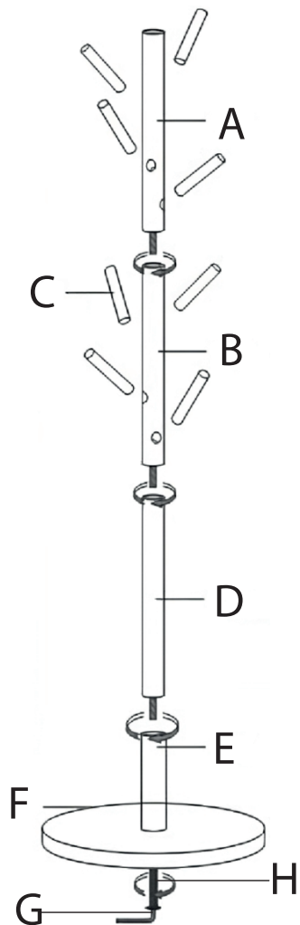
Схема сборки
